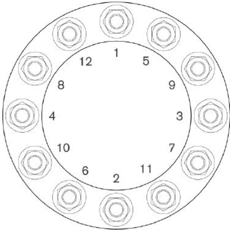
12 Stud Bolt Pattern
