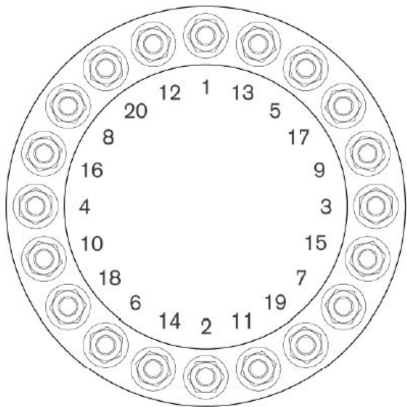
20 Stud Bolt Pattern
