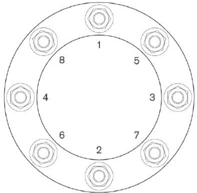
8 Stud Bolt Pattern
