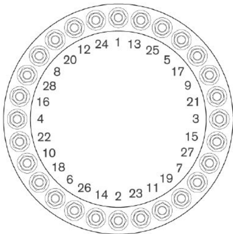
28 Stud Bolt Pattern
