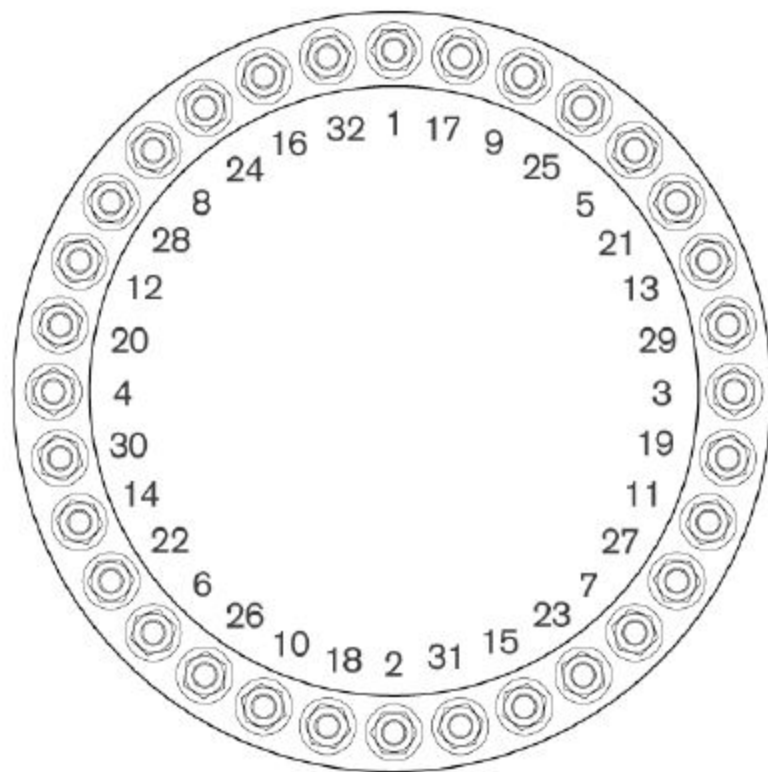
32 Stud Bolt Pattern
