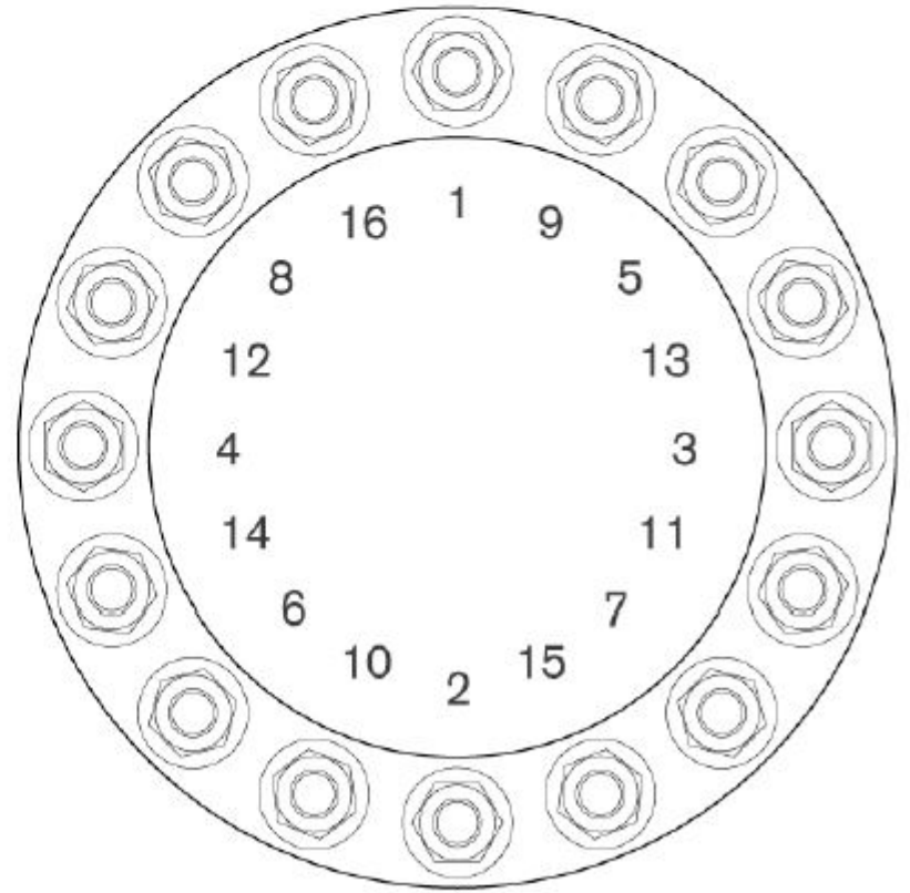
16 Stud Bolt Pattern
