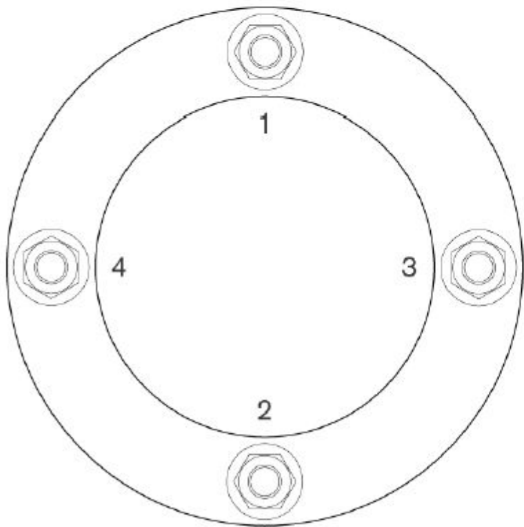
4 Stud Bolt Pattern
