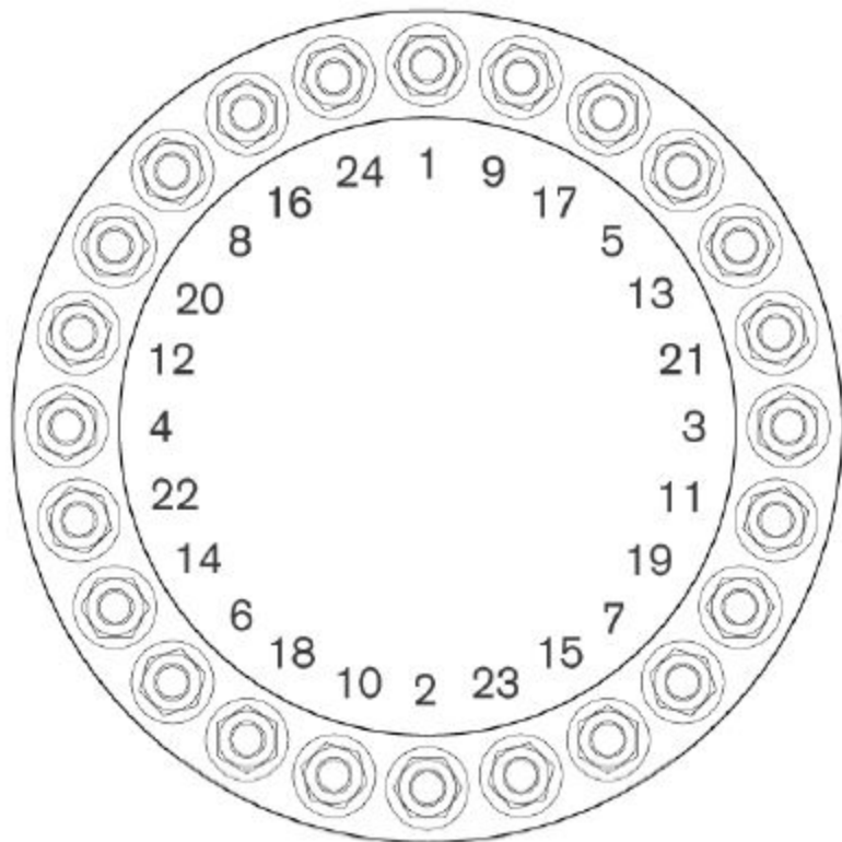
24 Stud Bolt Pattern
